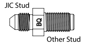
BQ157 -3 JIC to 1/8-28 BSPP
