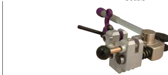
37° or 45° Double Bubble DIN
